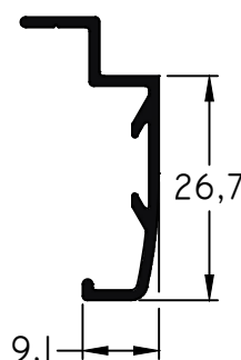
863 - Contramarco de atornillar Largo Std.: 6150 mm peso: 0,21 Kg/m
