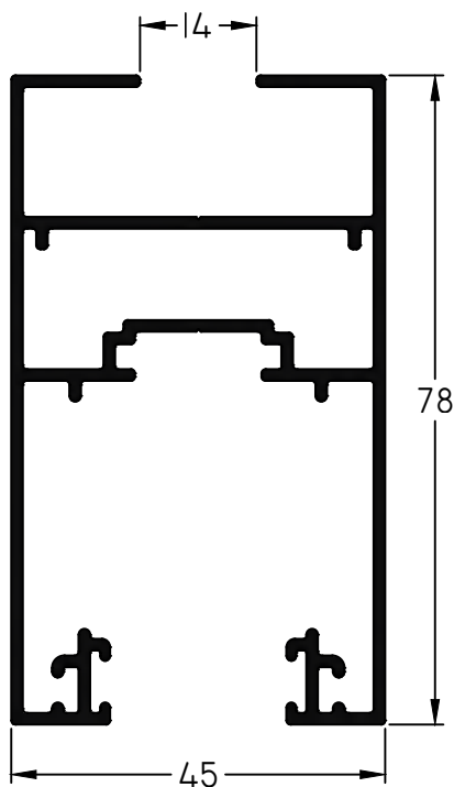
409 - Hoja Corrediza 45° VS Largo Std.: 6150 mm peso: 1,34 Kg/m
