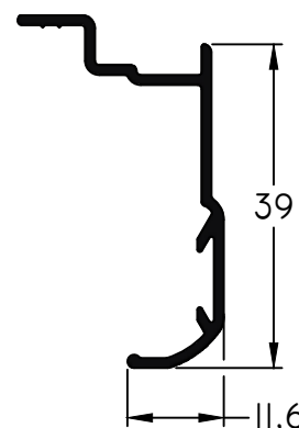
152 - Contramarco de atornillar Largo std.: 6150 mm Peso: 0,26 Kg/m
