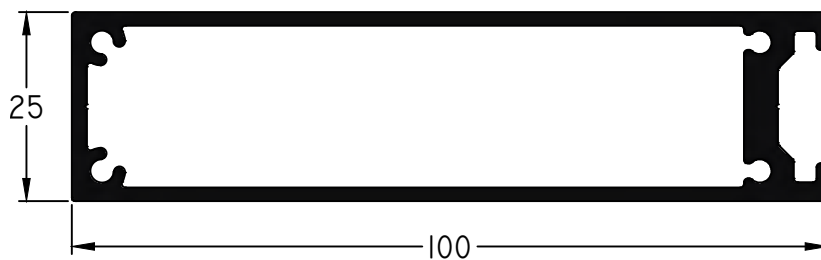
999 - Refuerzo inercial 100 mm Largo Std.: 6150 mm peso: 1,45 Kg/m
