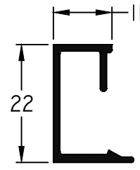
053 - Contravidrio recto 11 mm para clip Largo Std.: 6030 mm peso: 0,19 Kg/m
