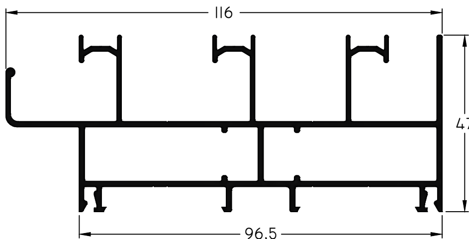
404 - Marco corrediza dos guías Largo Std.: 6150 mm peso: 1,16 Kg/m
