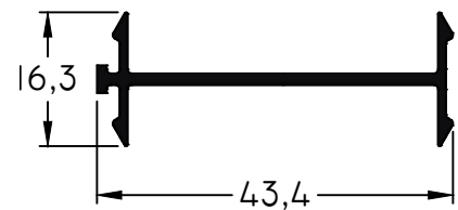
720 - Acople Largo Std.: 6150 mm peso: 0,26 Kg/m
