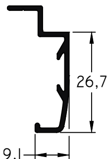
863 - Contramarco peso: 0,21 Kg/m
