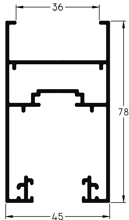
410 - Hoja Corrediza 45° DVH Largo Std.: 6150 mm peso: 1,26 Kg/m
