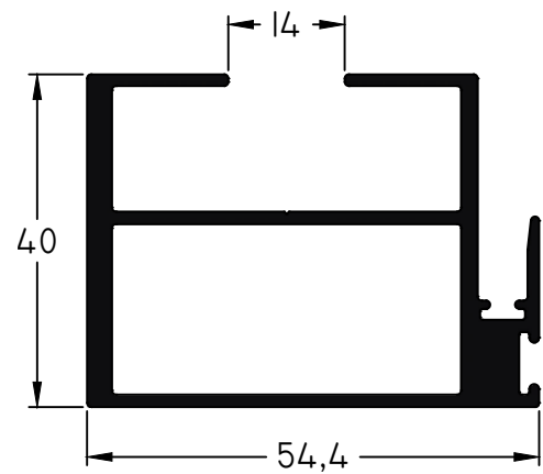
744 - Parante central hoja corte 90° VS Largo Std.: 6150 mm peso: 1,21 Kg/m
