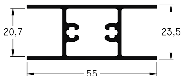
681 - Travesaño para Hoja N-Uno Largo Std.: 6030 mm peso: 0,70 Kg/m
