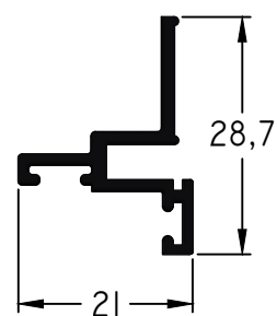
725 - Tope Inferior Umbral Largo Std.: 6030 mm peso: 0,26 Kg/m
