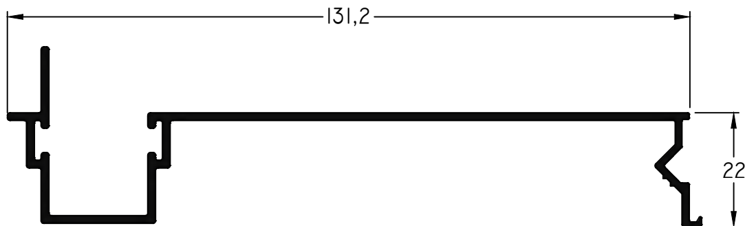
684 - Guía Barrio Largo Std.: 6150 mm peso: 0,89 Kg/m
