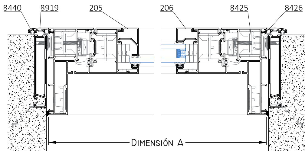
A-A Corte Horizontal
