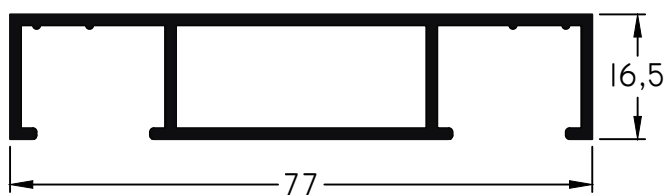
715 - Premarco Largo Std.: 6150 mm Peso: 0,70 Kg/m
