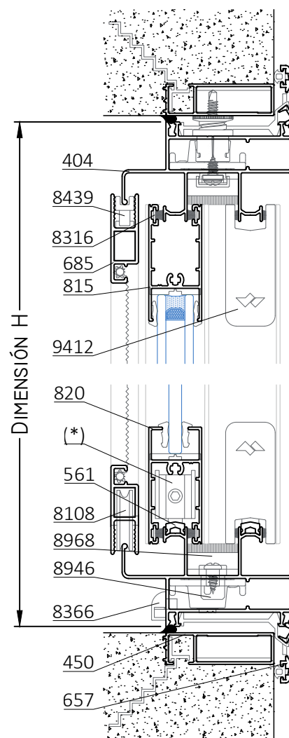
B-B Corte Vertical
