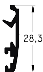
657 - Contramarco Largo Std.: 6150 mm peso: 0,19 Kg/m
