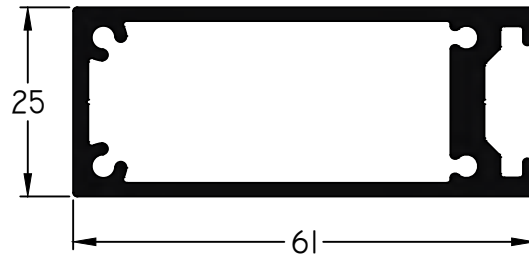
998 - Refuerzo inercial 61 mm Largo Std.: 6150 mm peso: 1,08 Kg/m
