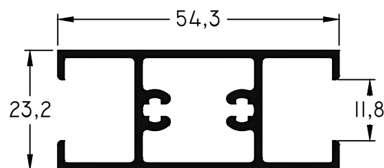
638 - Travesaño para hoja N-Uno Largo Std.: 6030 mm peso: 0,70 Kg/m
