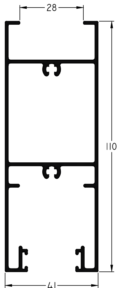
728 - Zócalo alto hoja 90° DVH 28 mm Largo Std.: 6030 mm peso: 1,49 Kg/m
