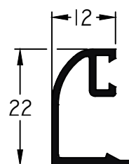
195 - Contravidrio curvo 12 mm Largo Std.: 6030 mm peso: 0,19 Kg/m
