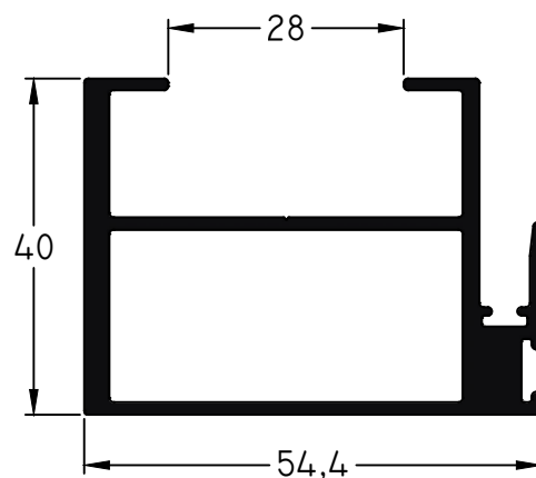
717 - Parante cent hoja 90° DVH 28 mm Largo Std.: 6150 mm peso: 1,16 Kg/m
