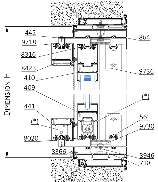
B-B Corte Vertical
