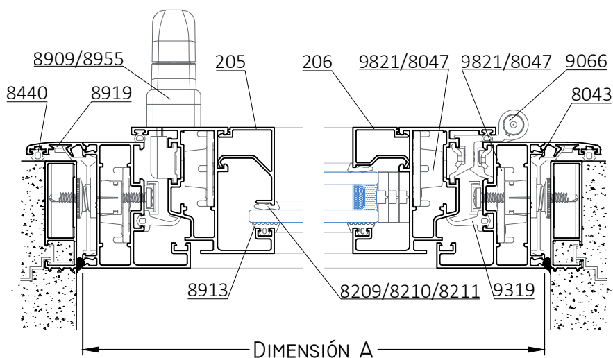
A-A Corte Horizontal
