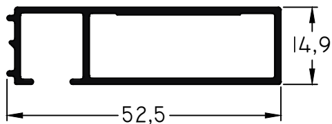
450 - Premarco 52 mm largo Std.: 6150 mm peso: 0,45 Kg/m
