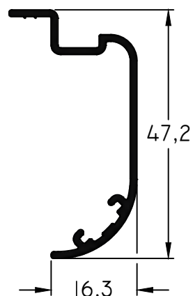
641 - Contramarco peso: 0,32 Kg/m
