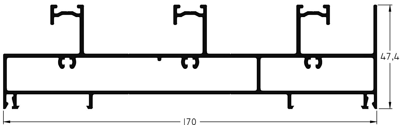
793 - Umbral Dintel 3 guías Largo Std.: 6150 mm peso: 2,54 Kg/m
