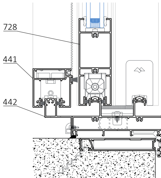
A-A Corte Horizontal
