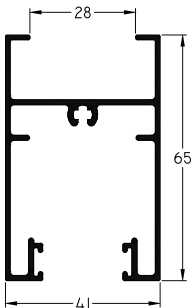
724 - Zócalo /cabezal hoja 90° DVH 28 mm Largo Std.: 6030 mm peso: 0,91 Kg/m
