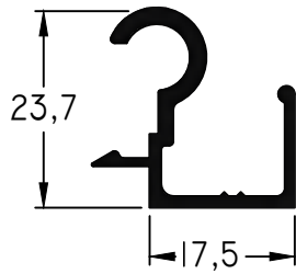
682 - Bisagra Tapacinta Largo Std.: 6150 mm peso: 0,27 Kg/m
