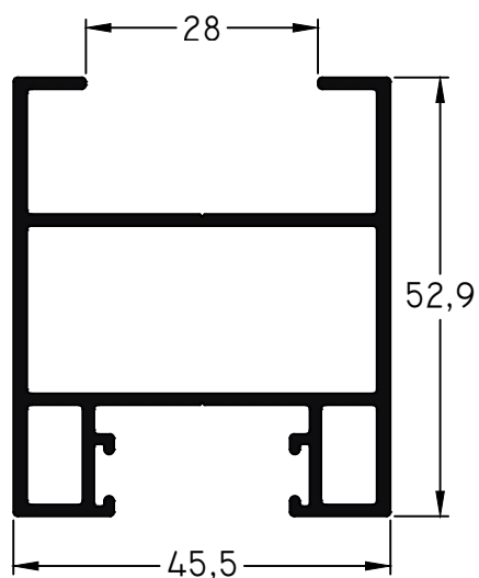
716 - Parante lat hoja 90° DVH 28 mm Largo Std.: 6150 mm peso: 1,04 Kg/m
