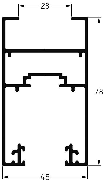
467 - Hoja Corrediza 45° DVH 28 mm Largo Std.: 6150 mm peso: 1,29 Kg/m
