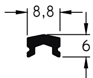
561 - Guía Inferior Corrediza Largo Std.: 6030 mm peso: 0,09 Kg/m
