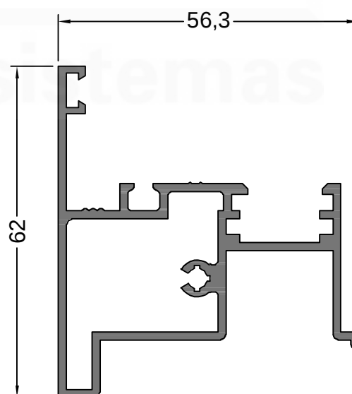
13211 1.076 Kg/m PUERTA ENCUESTRO 2 HOJAS
