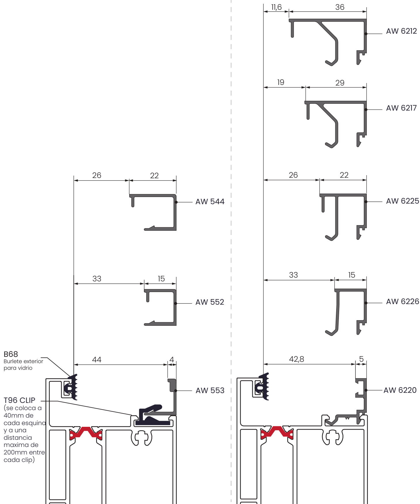
CONTRAVIDRIOS CORTE A 45°
