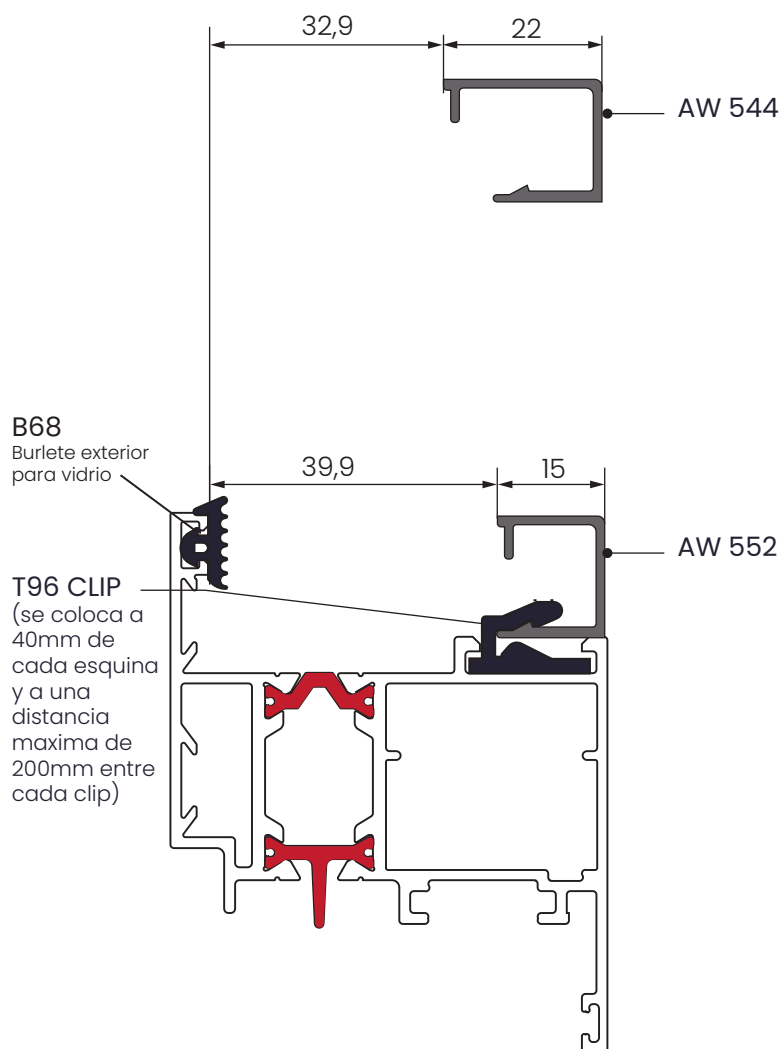
CONTRAVIDRIOS CORTE A 45°
