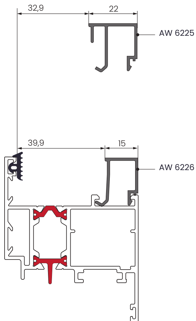
CONTRAVIDRIOS CORTE A 90°
