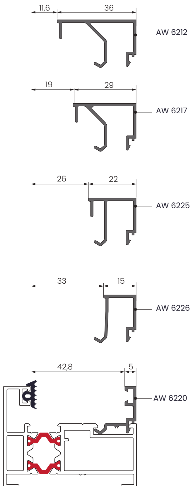
CONTRAVIDRIOS CORTE A 90°
